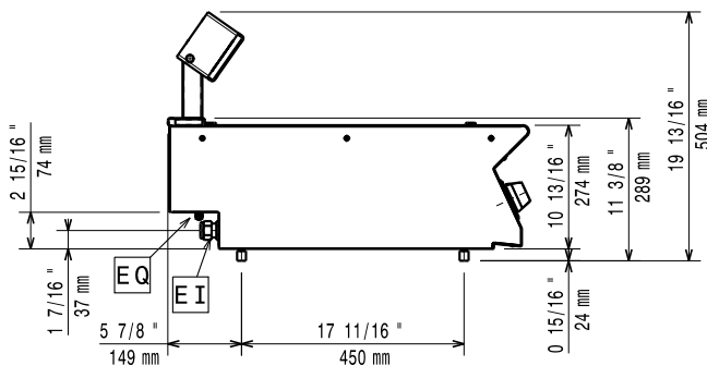
Zij aanzicht
